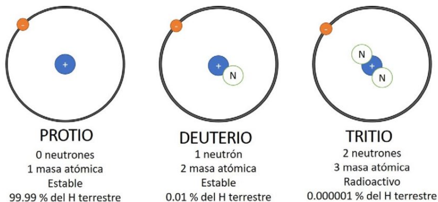
Figure 1: Isótopos hidrógeno
